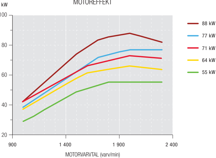
MF 3 SPECIALISTSERIE – MOTOREFFEKT & VRIDMOMENT
