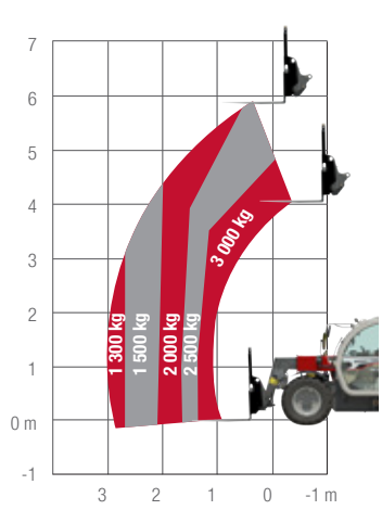
MF TH.6030
