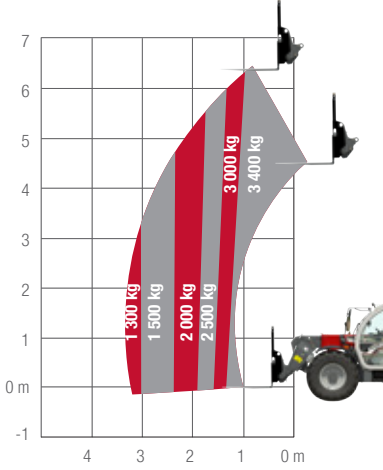
MF TH.6534
