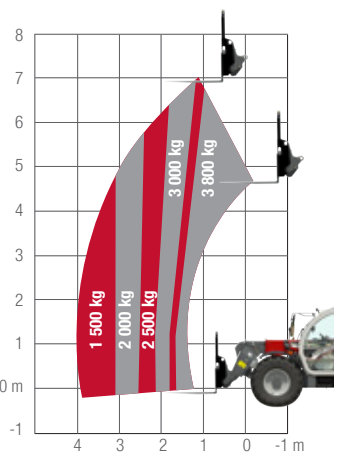
MF TH.7038
