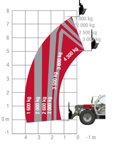
MF TH.8043
