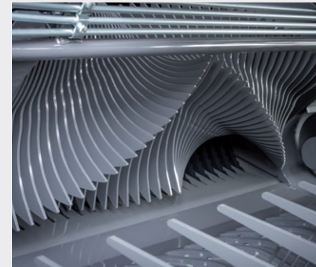
▲ Xtracut 25-rotoren har en spiraldesign med fire kniver som gir ekstrem kutteytelse.
