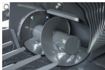
▲ INDFØRINGSSNEGLE
