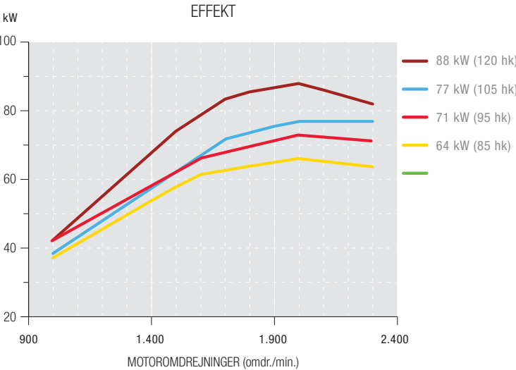
MF 3 SPECIALITY-SERIEN – MOTORKRAFT OG MOMENTKURVER
